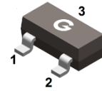
SOT-23-3L
